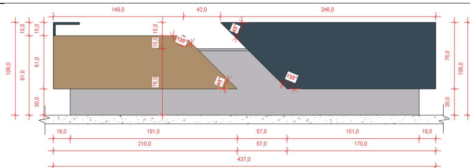
Vista frontal – 01
