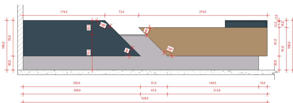
Vista frontal - 02
