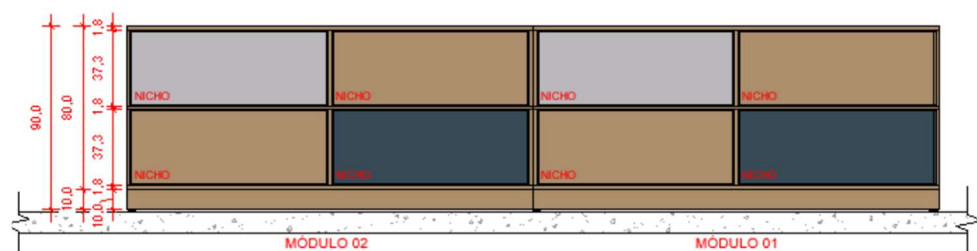
2 VISTA FRONTAL - FACE B 1 : 25 *MEDIDAS EM CENTÍMETROS
