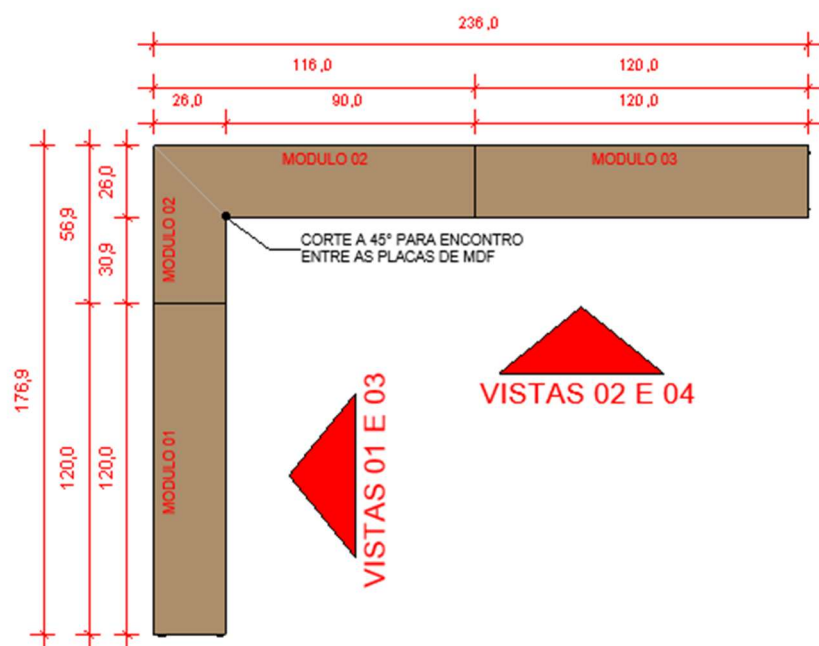
1 VISTA SUPERIOR 1:25 *MEDIDAS EM CENTIMETROS
