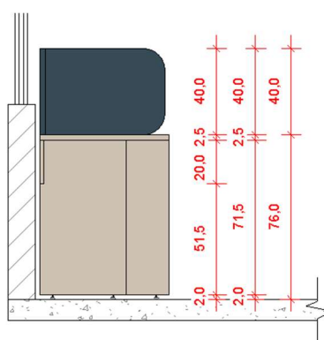
6 CORTE 1 : 25 *MEDIDAS EM CENTIMETROS
