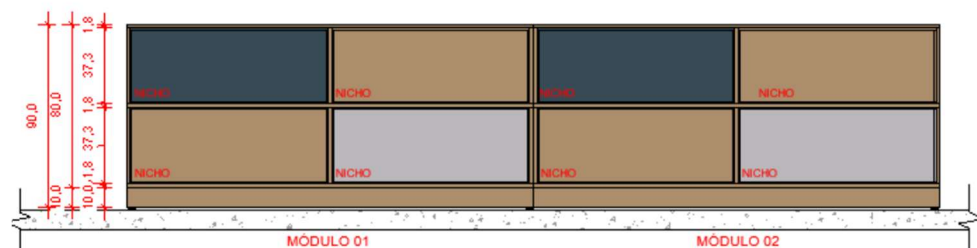
1 VISTA FRONTAL - FACE A 1 : 25 *MEDIDAS EM CENTÍMETROS
