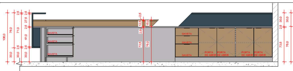
5 VISTA INTERNA 02 1:25 *MEDIDAS EM CENTIMETROS
