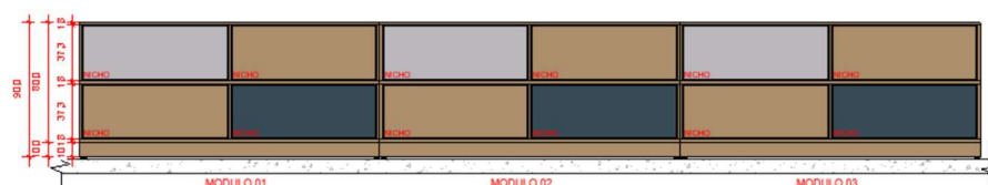
1 VISTA FRONTAL - FACE A 1:25 *MEDIDAS EM CENTÍMETROS
