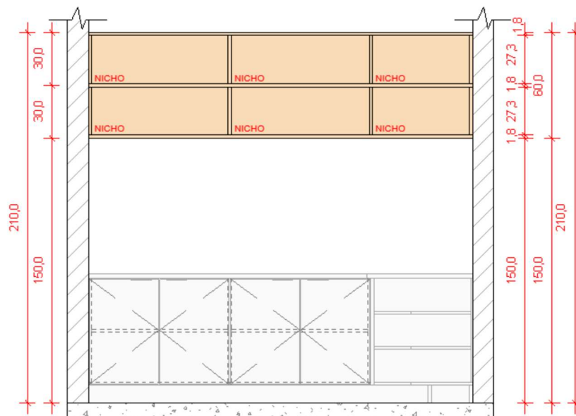
5 VISTA FRONTAL - CONJUNTO SUPERIOR 1 : 25 *MEDIDAS EM CENTÍMETROS
