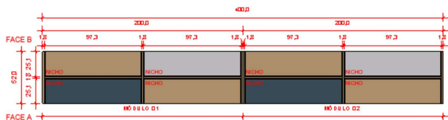
3 VISTA SUPERIOR 1 : 25 *MEDIDAS EM CENTÍMETROS
