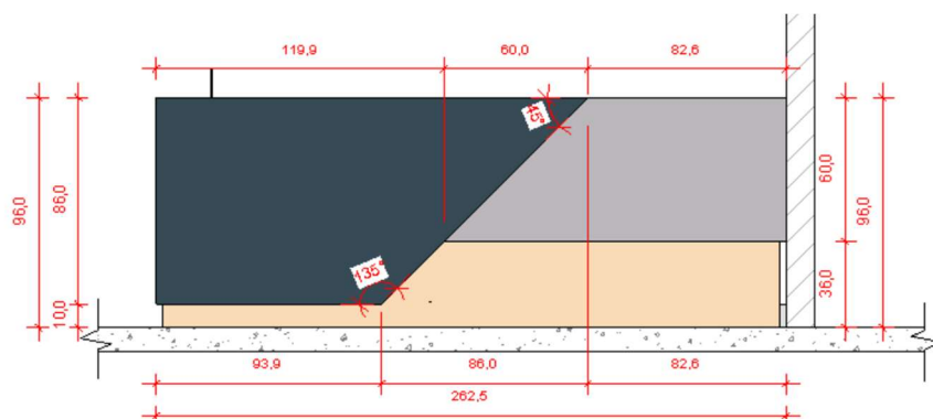
2 VISTA LATERAL 1:25 *MEDIDAS EM CENTIMETROS
