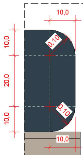
Detalhe quina arredondada
