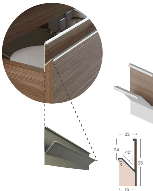
Vistas de detalhe – puxador perfil “cava”
