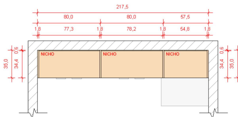
6 PLANTA BAIXA SUPERIOR 1 : 25 *MEDIDAS EM CENTÍMETROS
