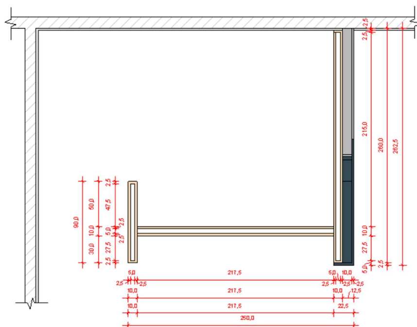
8 PLANTA BAIXA INFERIOR 1:25 *MEDIDAS EM CENTÍMETROS
