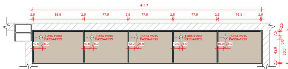
3 VISTA SUPERIOR 1 : 25 *MEDIDAS EM CENTIMETROS
