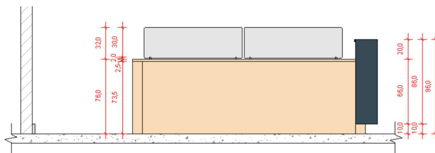
1 VISTA FRONTAL 1:25 *MEDIDAS EM CENTIMETROS
