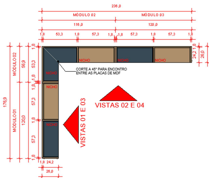
2 PLANTA BAIXA 1:25 *MEDIDAS EM CENTIMETROS
