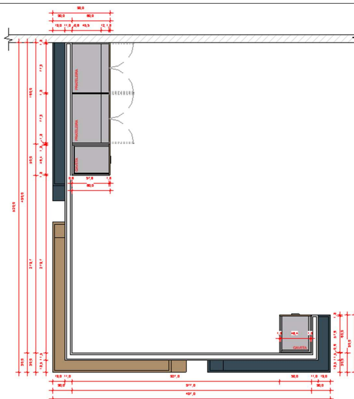
8 PLANTA BAIXA INFERIOR 1:25 MEDIDAS EM CENTÍMETROS
