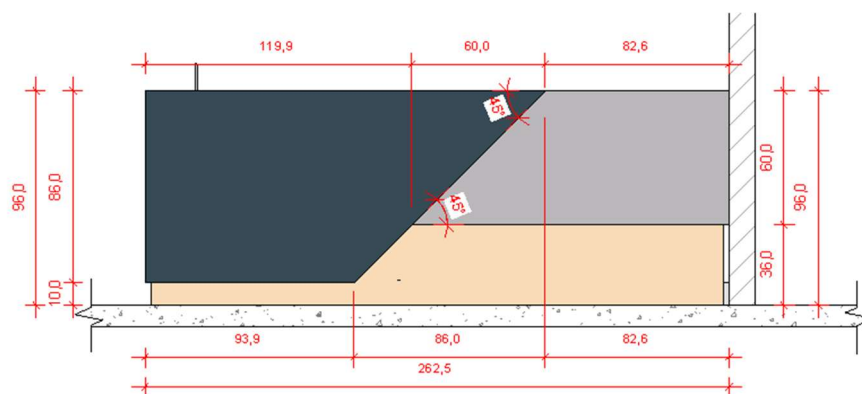
Vista frontal - painéis
