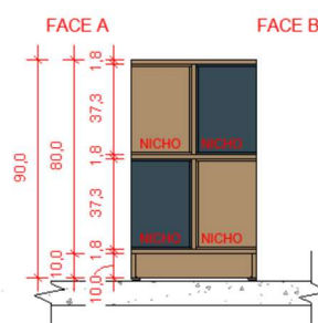
6 CORTE AA 1:25 *MEDIDAS EM CENTÍMETROS
