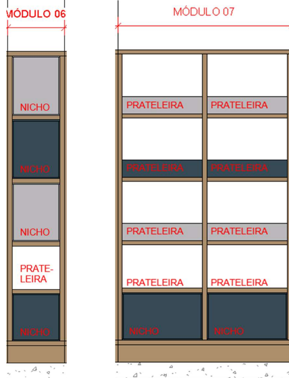
Vistas frontais
