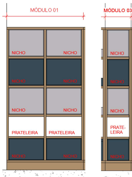
Vistas frontais
