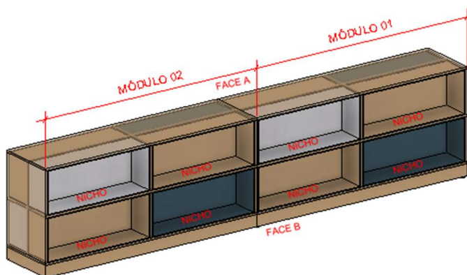
Perspectiva – Face B
