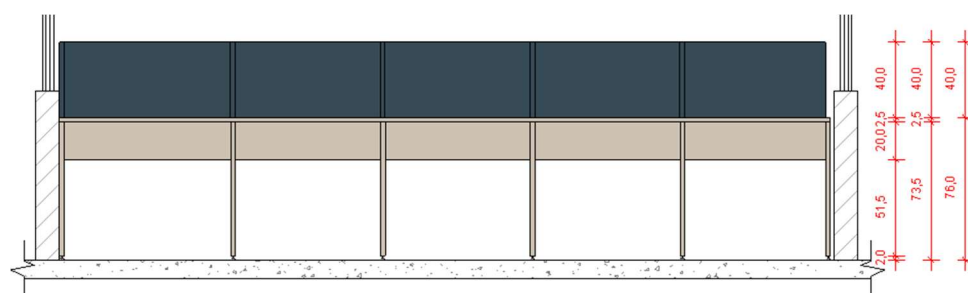
5 VISTA FRONTAL 1 : 25 *MEDIDAS EM CENTIMETROS
