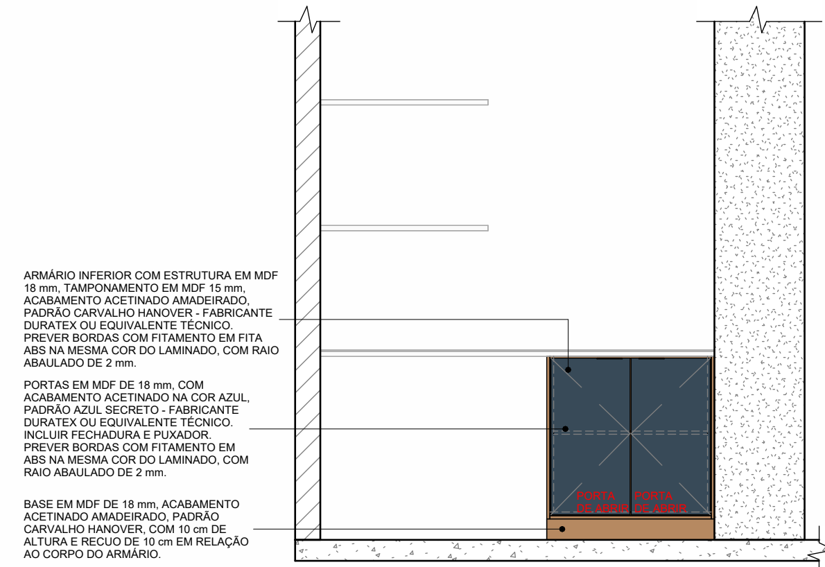
12 VISTA FRONTAL - ARMÁRIO 1:25 *MEDIDAS EM CENTÍMETROS
