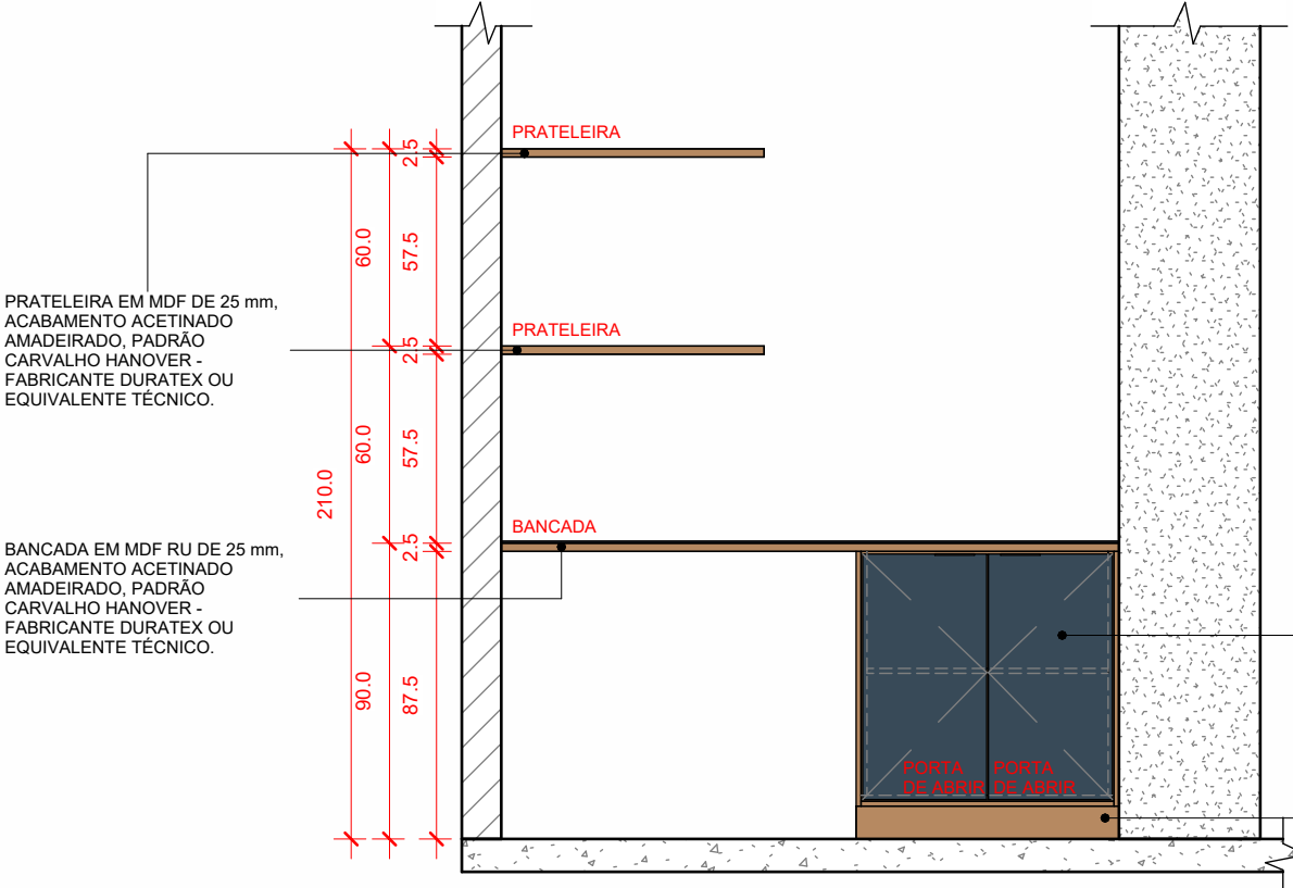
1 VISTA FRONTAL - GERAL 1:25 *MEDIDAS EM CENTÍMETROS
