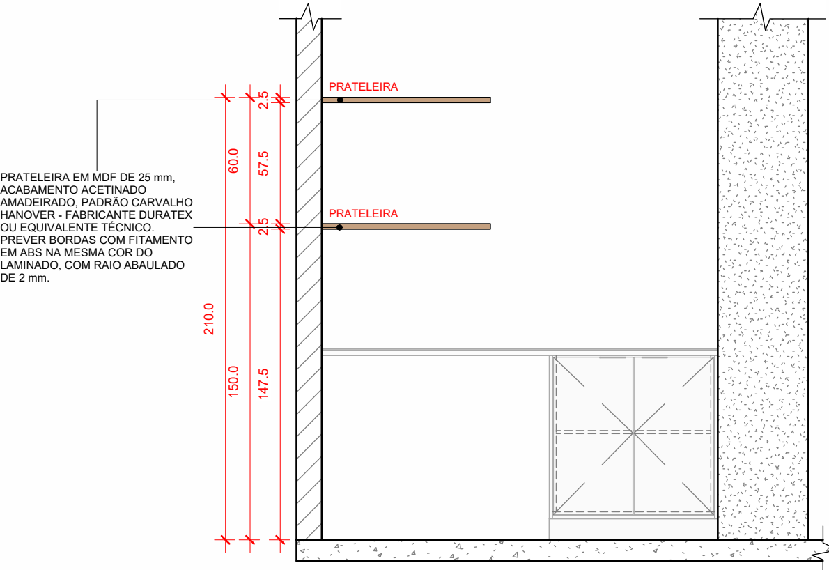
4 VISTA FRONTAL - PRATELEIRAS 1:25 *MEDIDAS EM CENTÍMETROS
