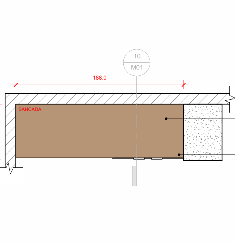
9 PLANTA BAIXA - BANCADA 1:25 *MEDIDAS EM CENTÍMETROS
