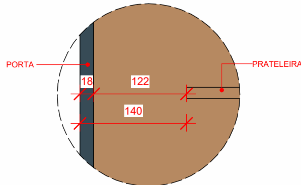
16 DET. 01 1:5 *MEDIDAS EM MILÍMETROS
