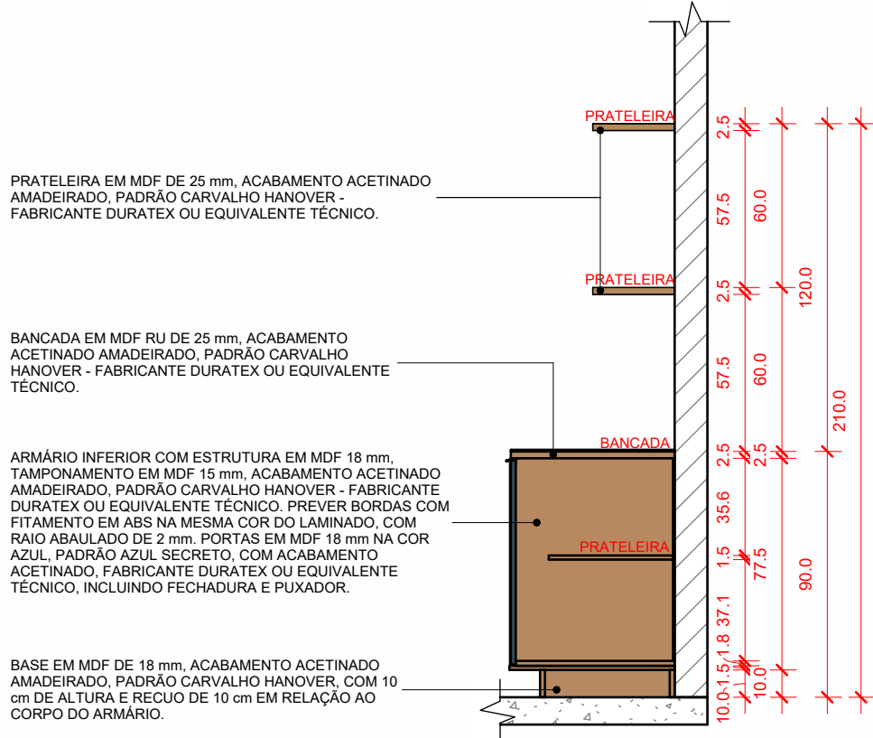
2 CORTE GERAL 1:25 *MEDIDAS EM CENTÍMETROS
