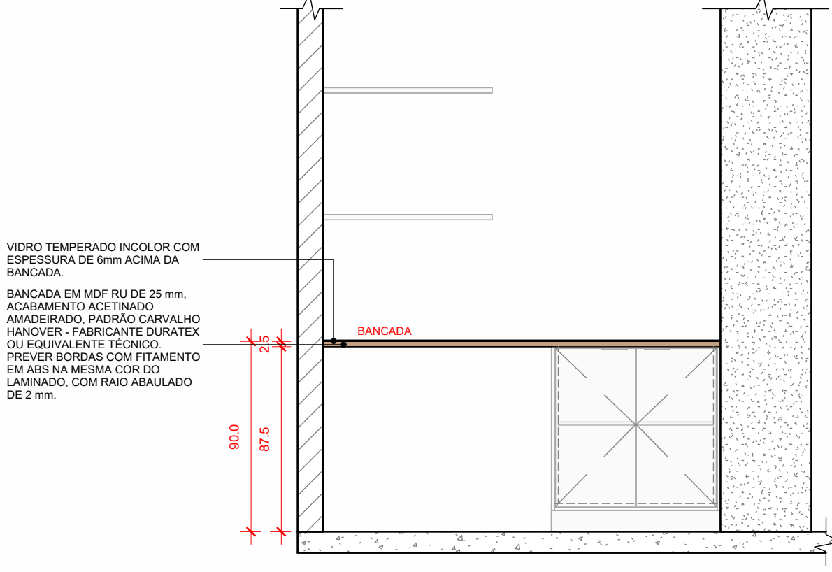
8 VISTA FRONTAL - BANCADA 1:25 *MEDIDAS EM CENTÍMETROS
