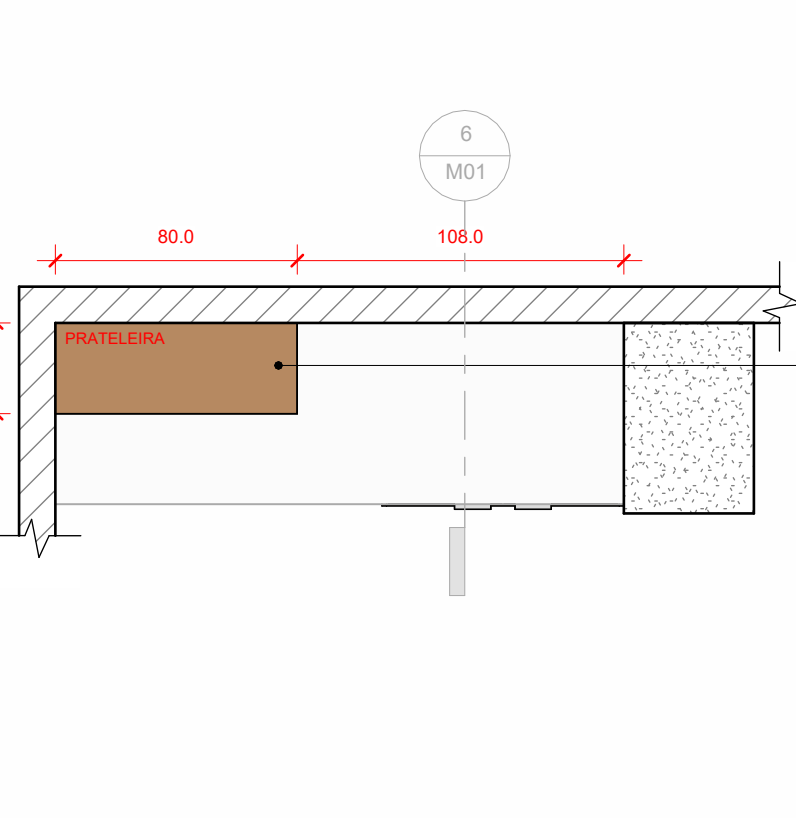
5 PLANTA BAIXA - PRATELEIRAS 1:25 *MEDIDAS EM CENTÍMETROS
