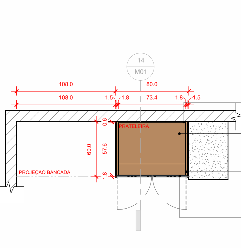
13 PLANTA BAIXA - ARMÁRIO 1:25 *MEDIDAS EM CENTÍMETROS
